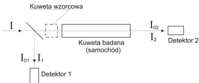
Rys. 6. Schemat układu badawczego wykorzystującego metodę porównawczą
