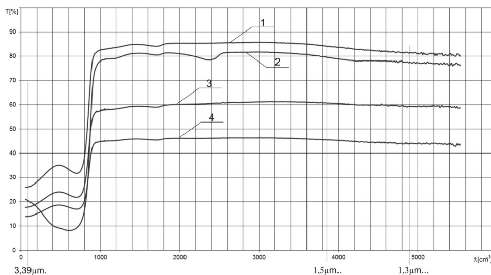
Rys. 2. Transmisja promieniowania przez płytki szklane w funkcji liczby falowej dla: 1 – płytki czystej, 2 – „zaparowanej” parą wodną, 3 – pokrytej pyłem z gleby, 4 – pokrytej pyłem grafitowym
