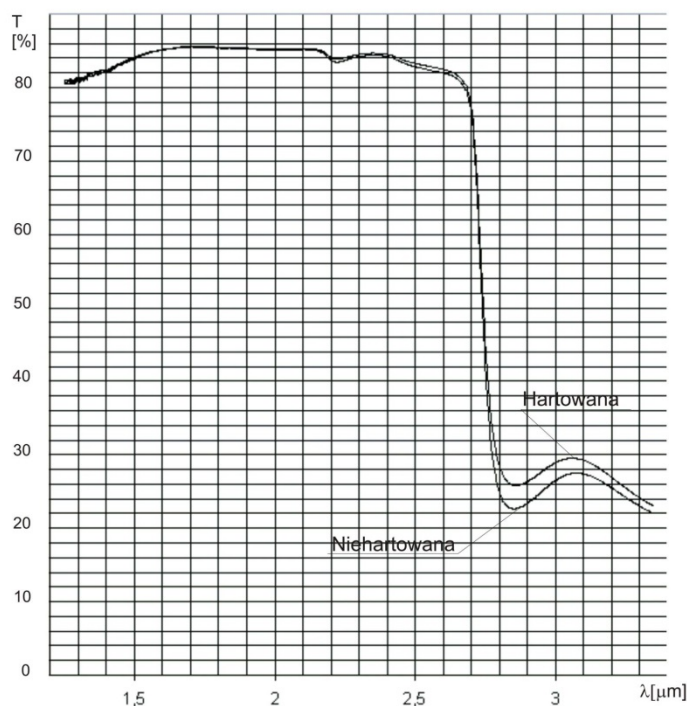
Rys. 3. Transmisja hartowanej i niehartowanej szyby bocznej samochodu w funkcji długości fali promieniowania prześwietlającego.
