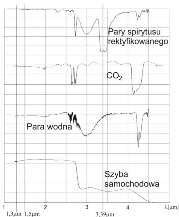
Rys. 1. Zestawienie charakterystyk spektralnych substancji mogących występować w sprawdzanym samochodzie
