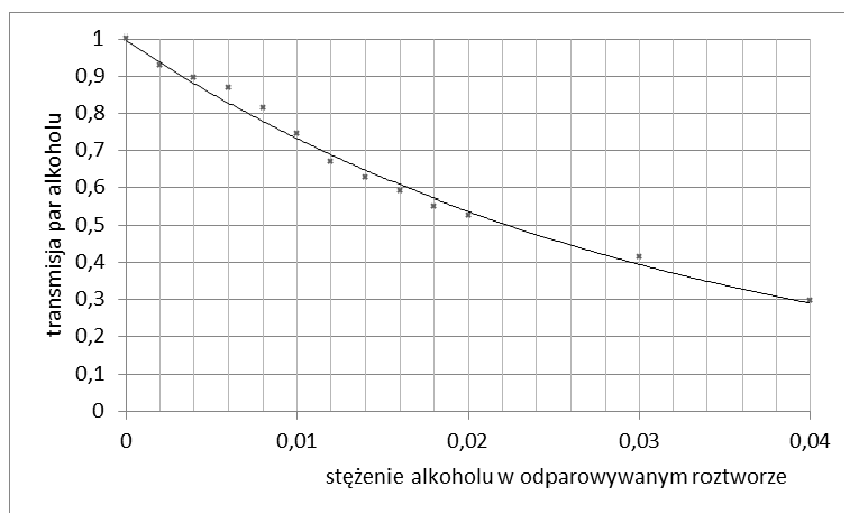
Rys. 10. Wykres transmisji par alkoholu w funkcji stężenia w parującym roztworze
