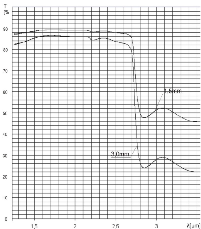
Rys. 4. Wyniki pomiarów na spektrofotometrze płytek ze szkła flot o grubościach 1,5 mm i 3,0 mm
