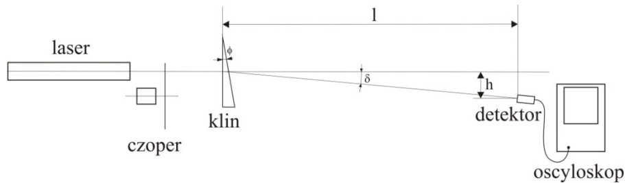
Rys. 5. Schemat układu eksperymentalnego do pomiaru współczynnika załamania szkła
