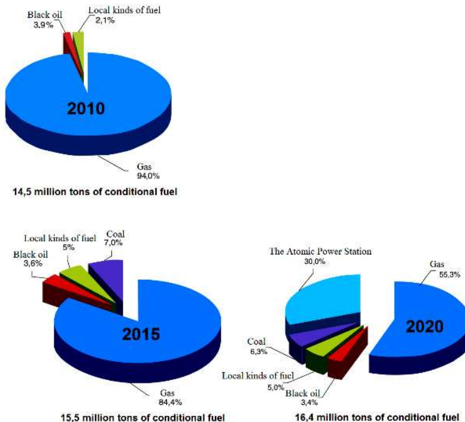
Рис. 3. Структура топливного баланса Белорусской энергосистемы на 2010, 2015 и 2020 гг. Fig. 3. Structure of fuel balance of the Belarus power supply system in 2010, 2015 and 2020
