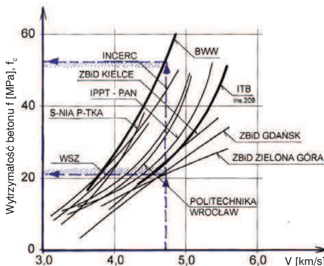
Rys. 4. Przykłady charakterystycznych zależności f_c - V dla metody ultradźwiękowej
