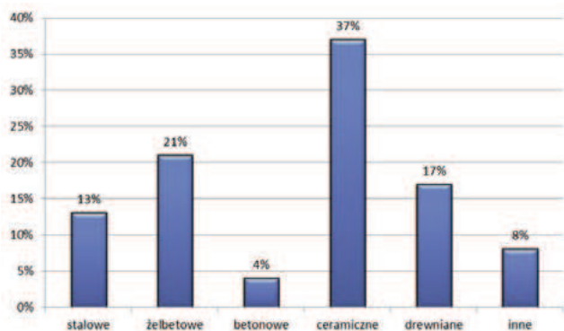
Rys. 3. Udział procentowy awarii i katastrof w latach 1962–2013 według podziału ze względu na materiały
