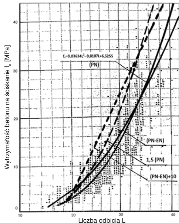
Rys. 6. Zależności empiryczne dla młotków Schmitta typu N ( \alpha=0 ) do oceny wytrzymałości betonu podane dla warunków polskich [7]
