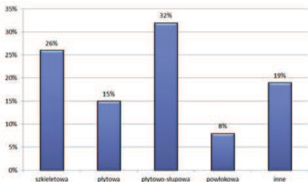
Rys. 2. Udział procentowy awarii i katastrof w latach 1962–2013, według podziału na typy konstrukcji budowlanych
