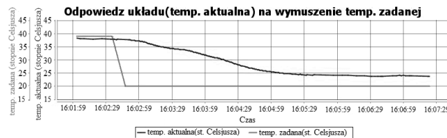
Rys. 5. Przebiegi temperatury mierzonej i zadanej przy wymuszeniu skokowym (chłodzenie) [4]
