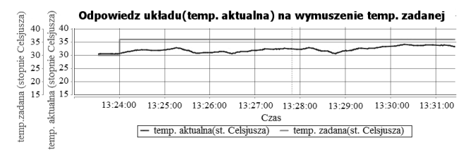
Rys. 10. Przebieg temperatury mierzonej po wymuszeniu zadana (grzanie) dla metody mieszania powietrza z regulatorem PID (dla k_p=25 ; T_i=2,5 ; T_d=10 , T_I=5 ) [4]
