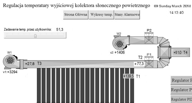
Rys. 13. Okno strony głównej tablicy synoptycznej zrealizowanej w Control Maestro [4]
