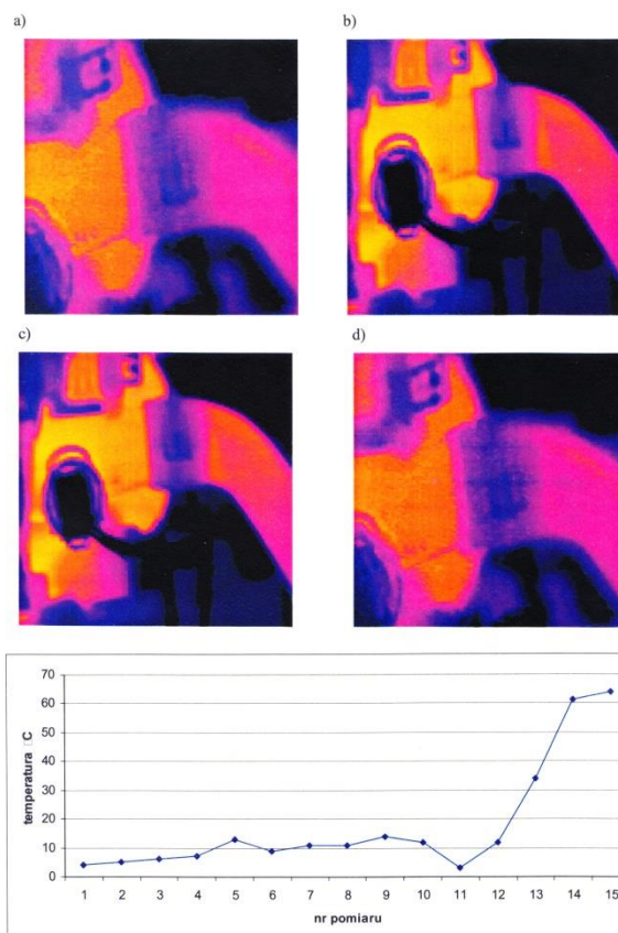
Rys. 3. Obrazy z kamery termowizyjnej dolnego wyjścia gumowego przewodu chłodniczego na silnik oraz wykres zależności temperatury od czasu działania silnika: a- przed rozruchem, b- 360 s po rozruchu, c-720s po rozruchu, d- 3480 s po rozruchu
