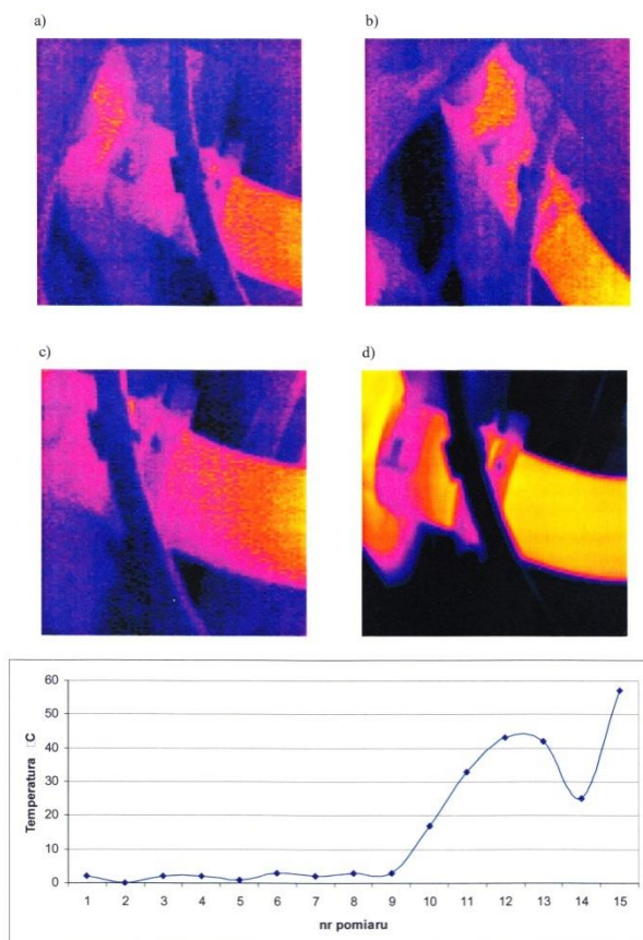
Rys. 2. Obrazy termalne górnego wejścia przewodu chłodniczego na chłodnicy gumowego przewodu chłodniczego przy silniku oraz wykres zależności temperatury od czasu działania silnika: a- przed rozruchem, b- 360 s po rozruchu, c-1080 s po rozruchu, d- 2760 s po rozruchu
