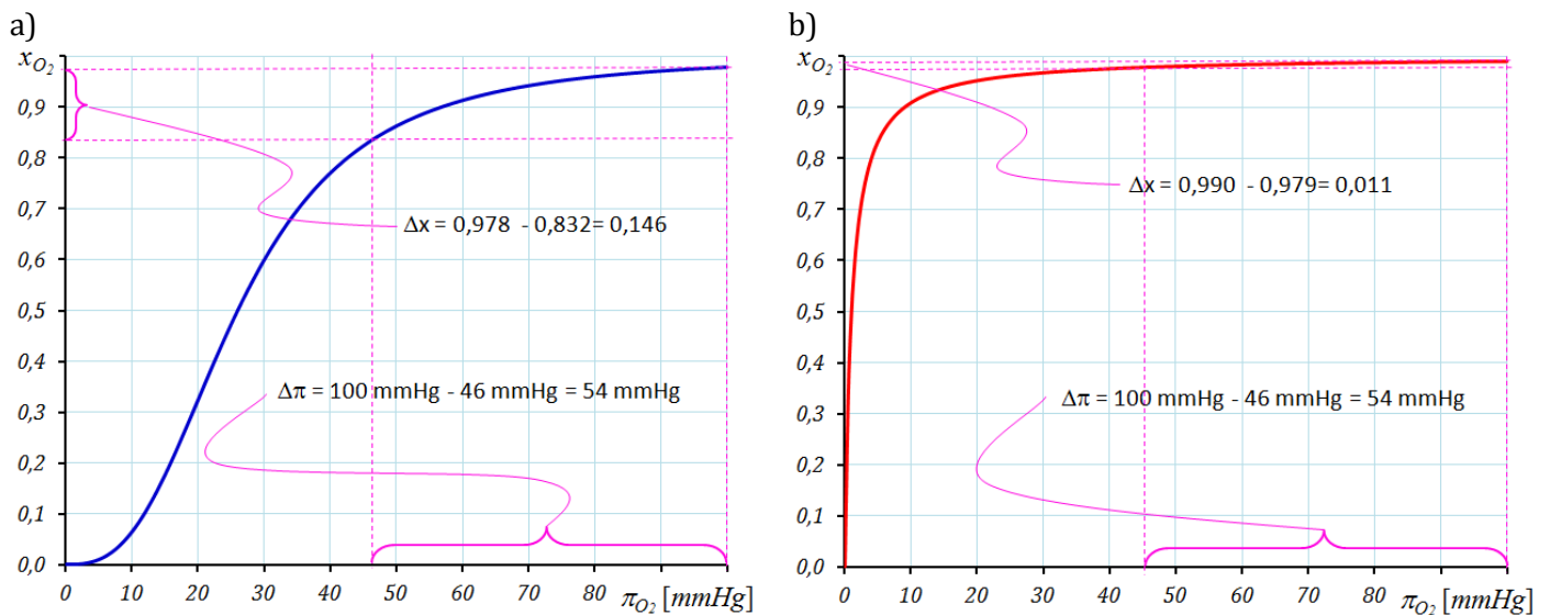
Rys. 3. Wykresy dysocjacji kompleksów a) hemoglobina-tlen , b) mioglobina-tlen jako zależność wysycenia tlenem x_{O_2} = \frac{[AO_2]}{[AO_2] + [A]} | A = \{Hb; Mb\} w funkcji prężności tlenu \pi_{O_2} we krwi przy założeniu, że ciśnienie cząstkowe tlenu w pęcherzykach płucnych będzie na poziomie p_{O_2} = 100 \text{ mmHg} a prężność tlenu w naczyniach włosowatych \pi_{O_2} = 46 \text{ mmHg} .
