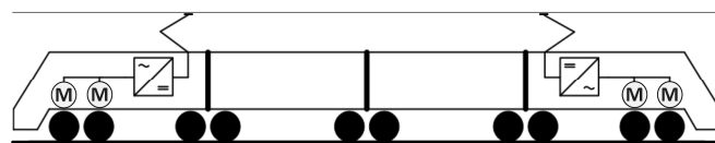
Rys. 1. Schemat blokowy układu napędowego ezt
