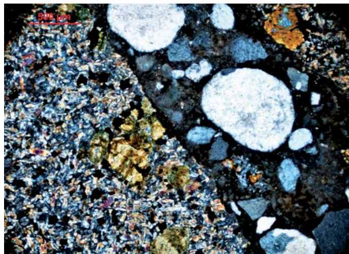
Fot. 17. Próbką 42/20 – dolna warstwa betonu; ziarna bazaltu – po lewej i prawy górny róg; obraz mikroskopowy w świetle przechodzącym spolaryzowanym (skrzyżowane polaryzatory) [7]
