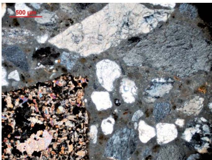
Fot. 8. Próbką 1118/19 – dolna warstwa betonu; widoczne ziarna piasku, żwiru i bazaltu (lewy dolny róg); obraz mikroskopowy w świetle przechodzącym spolaryzowanym (skrzyżowane polaryzatory) [7]
