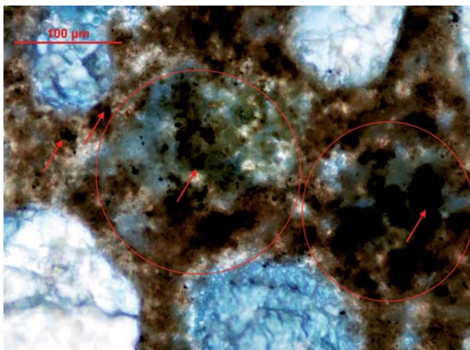
Fot. 20. Próbką 1118/19 – górna warstwa betonu; stwardniały zaczyn cementowy (brunatny) z relikami niezhydratyzowanych ziaren cementu (zaznaczone okręgami); widoczne liczne skupienia brownillerytu (czarne plamki i punkty zaznaczone strzałkami); obraz mikroskopowy w świetle przechodzącym spolaryzowanym (skrzyżowane polaryzatory) [7]
