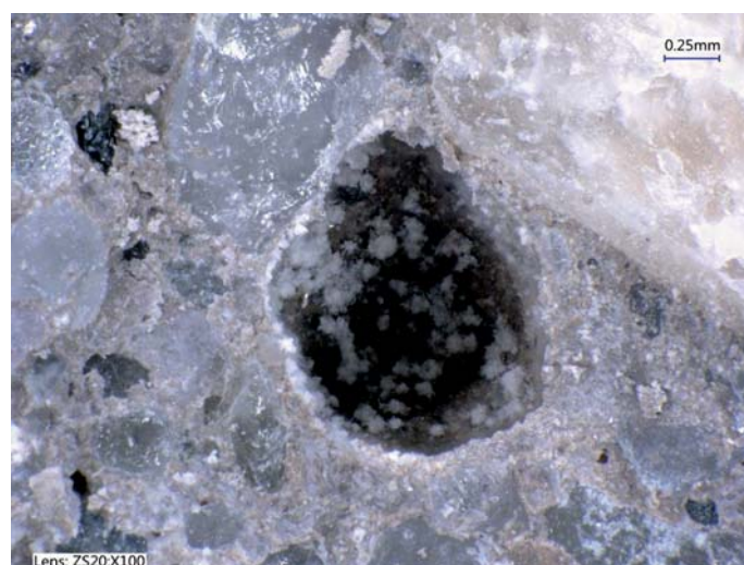
Fot. 28. Próbką 1118/19 – górna warstwa betonu, widoczny jest por powietrzny [7]
