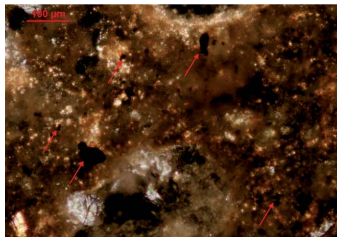
Fot. 23. Próbką 49/20 – dolna warstwa betonu; stwardniały zaczyn cementowy (brązowy) ze skupieniami czarnego brownillerytu (strzałki); obraz mikroskopowy w świetle przechodzącym spolaryzowanym (skrzyżowane polaryzatory) [7]
