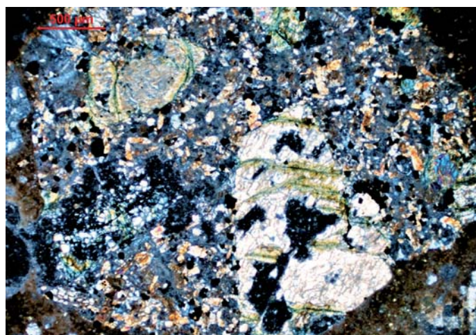
Fot. 19. Próbką 49/20 – górna warstwa betonu; ziarno bazaltu; widoczne fenokryształy oliwiny wtórnie przeobrażone w zielony bowlingit; obraz mikroskopowy w świetle przechodzącym spolaryzowanym (skrzyżowane polaryzatory) [7]
