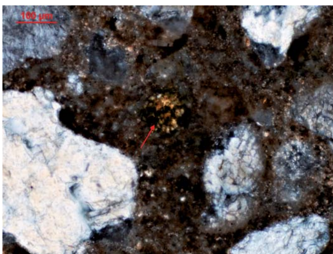
Fot. 21. Próbką 1118/19 – górna warstwa betonu; niezhydratyzowane ziarno cementu w stwardniałym zaczynie (zaznaczone strzałką); obraz mikroskopowy w świetle przechodzącym spolaryzowanym (skrzyżowane polaryzatory) [7]
