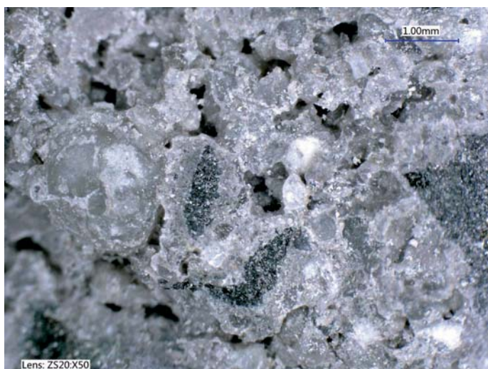
Fot. 31. Próbką 49/20 – dolna warstwa betonu, widoczna porowata struktura betonu [7]
