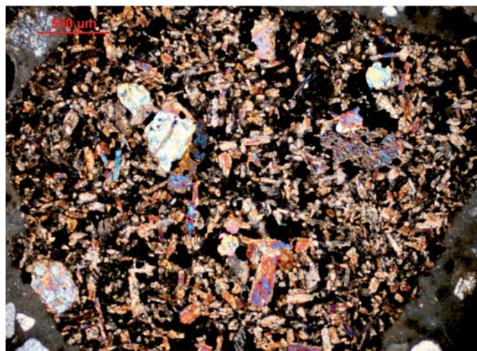
Fot. 18. Próbką 1118/19 – dolna warstwa betonu; ziarno bazaltu; obraz mikroskopowy w świetle przechodzącym spolaryzowanym (skrzyżowane polaryzatory) [7]
