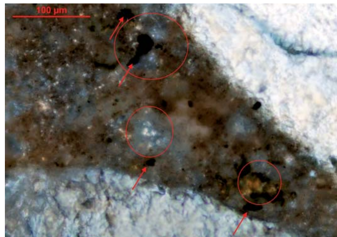
Fot. 22. Próbką 42/20 – górna warstwa betonu; stwardniały zaczyn cementowy (brązowy) z relikami niezhydratyzowanych ziaren cementu (okręgi) i skupieniami czarnego brownillerytu (strzałki); obraz mikroskopowy w świetle przechodzącym spolaryzowanym (skrzyżowane polaryzatory) [7]
