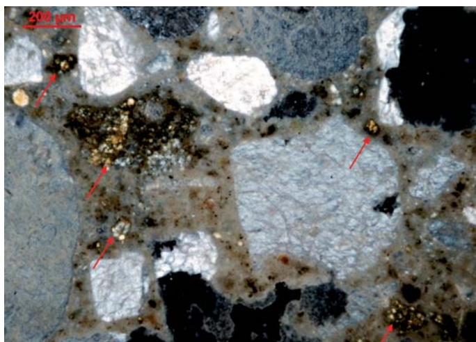
Fot. 26. Próbką 1124/19 – dolna warstwa betonu; stwardniały zaczyn cementowy z niezhydratyzowanymi ziarnami cementu (strzałki); obraz mikroskopowy w świetle przechodzącym spolaryzowanym (skrzyżowane polaryzatory) [7]
