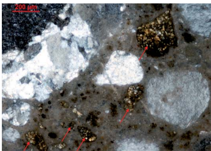
Fot. 27. Próbką 1124/19 – dolna warstwa betonu; stwardniały zaczyn cementowy z niezhydratyzowanymi ziarnami cementu (strzałki); obraz mikroskopowy w świetle przechodzącym spolaryzowanym (skrzyżowane polaryzatory) [7]
