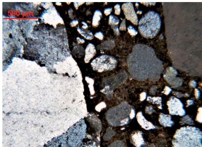
Fot. 9. Próbką 1124/19 – górna warstwa betonu; widoczne ziarna piasku i żwiru; obraz mikroskopowy w świetle przechodzącym spolaryzowanym (skrzyżowane polaryzatory) [7]
