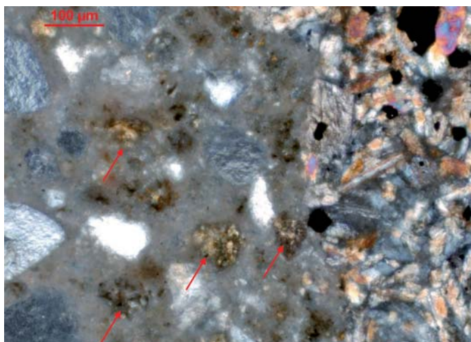
Fot. 25. Próbką 1118/19 – dolna warstwa betonu; stwardniały zaczyn cementowy z niezhydratyzowanymi ziarnami cementu (strzałki); obraz mikroskopowy w świetle przechodzącym spolaryzowanym (skrzyżowane polaryzatory) [7]
