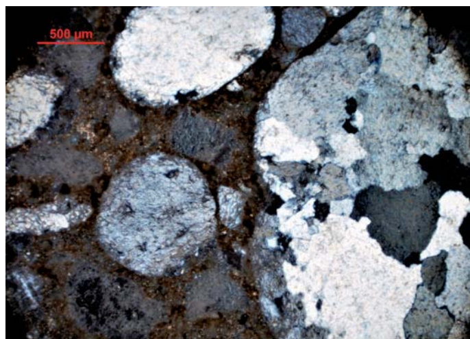
Fot. 11. Próbką 42/20 – górna warstwa betonu; widoczne ziarna piasku i żwiru; obraz mikroskopowy w świetle przechodzącym spolaryzowanym (skrzyżowane polaryzatory) [7]
