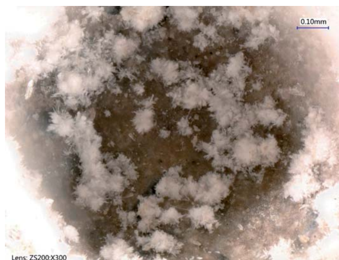
Fot. 29. Próbką 1118/19 – górna warstwa betonu, widoczny por powietrzny z mineralizacją (być może ettringit) na ściankach [7]
