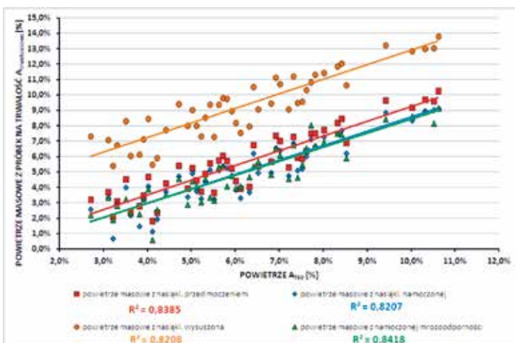
Rys. 4. Korelacja między zawartością powietrza A_{T60} a A_{twardziowe}
