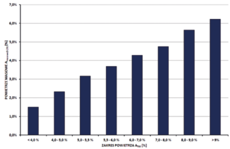
Rys. 5. Zależność w przedziałach zawartości powietrza A_{T60} a powietrzem masowym A_{masowe(fc28)}
