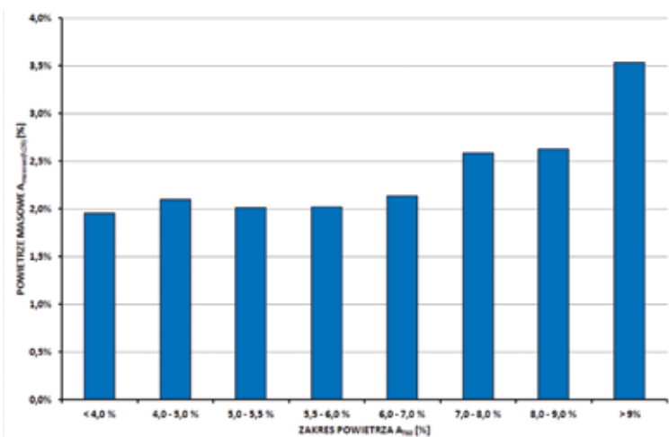
Rys. 6 Spadek zawartości powietrza masowego A_{masowe(fc28)} w przedziałach zawartości powietrza A_{T60}
