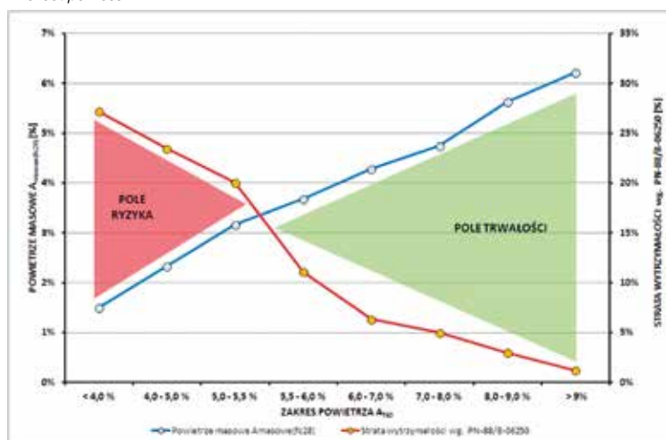
Rys. 9. Obszary określające ryzyko i ufność dla przedziałów zawartości powietrza określonych różnymi metodami w aspekcie straty wytrzymałości po badaniu mrozoodporności
