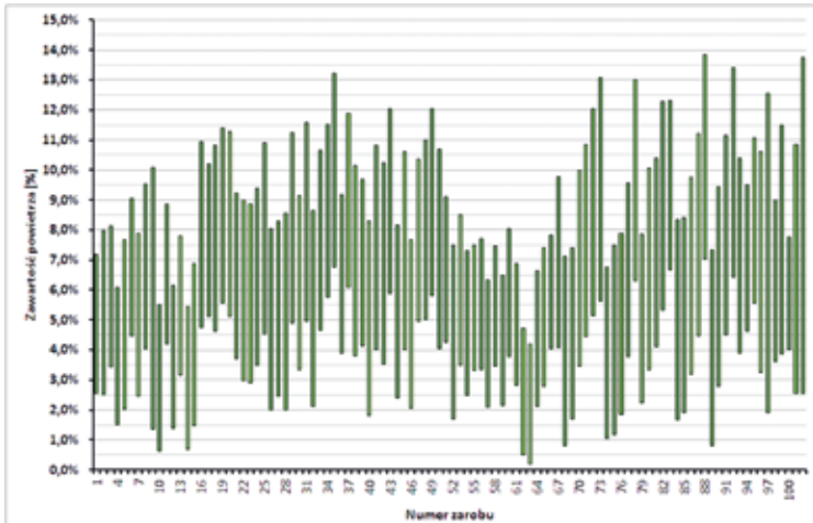
Rys. 2. Przedziały zawartości powietrza określone różnymi metodami dla poszczególnych zarobów
