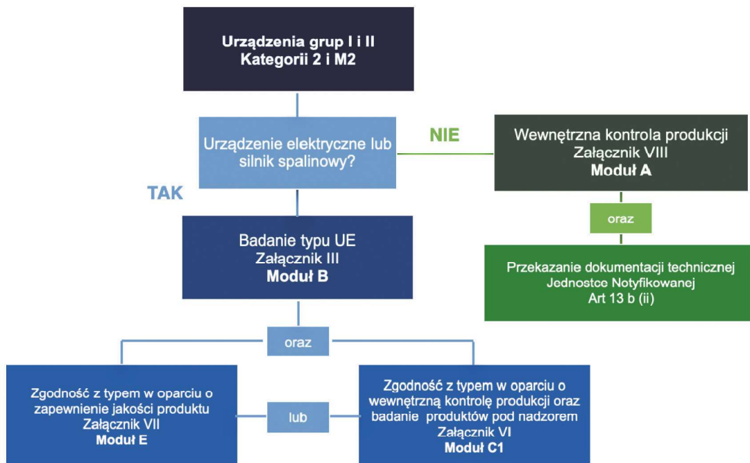
Rys. 6. Moduły oceny zgodności urządzeń kategorii M2
