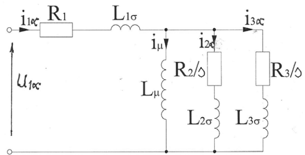
Rys. 3. Jednofazowy schemat zastępczy silnika przy pominięciu mocy strat w żelazie \Delta P_{fe} = 0
