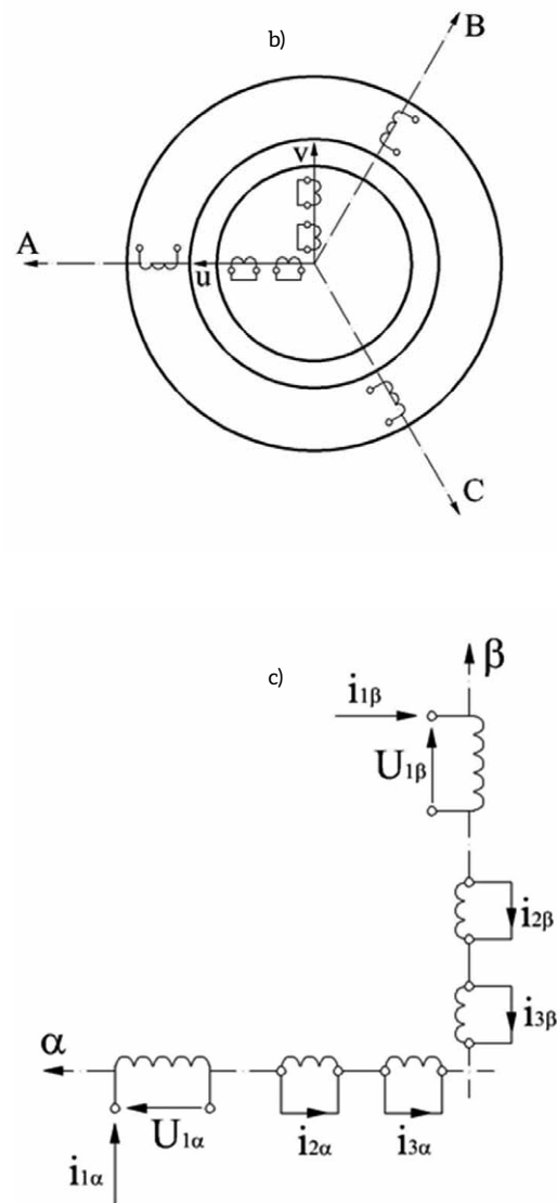
Rys. 2. Kolejne etapy transformacji uzwojeń silnika indukcyjnego klatkowego z układu trójfazowego do układu dwuosiowego \alpha, \beta : a – przekrój obwodu magnetycznego; b – schematyczne przedstawienie uzwojeń; c – uzwojenia w osiach \alpha, \beta nieruchomych względem stojana
