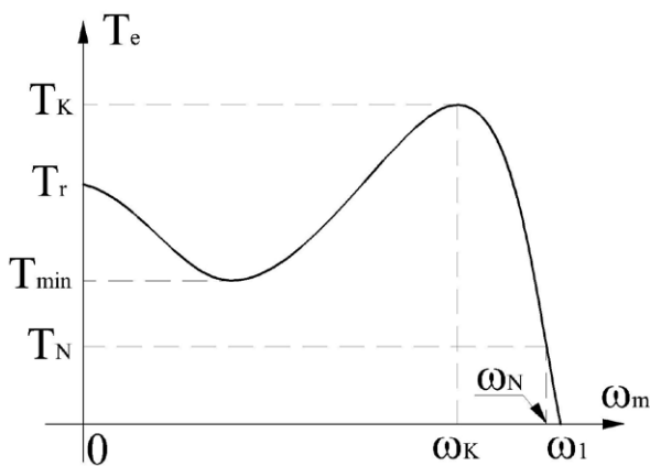
Rys. 1. Charakterystyka elektromechaniczna silnika indukcyjnego
