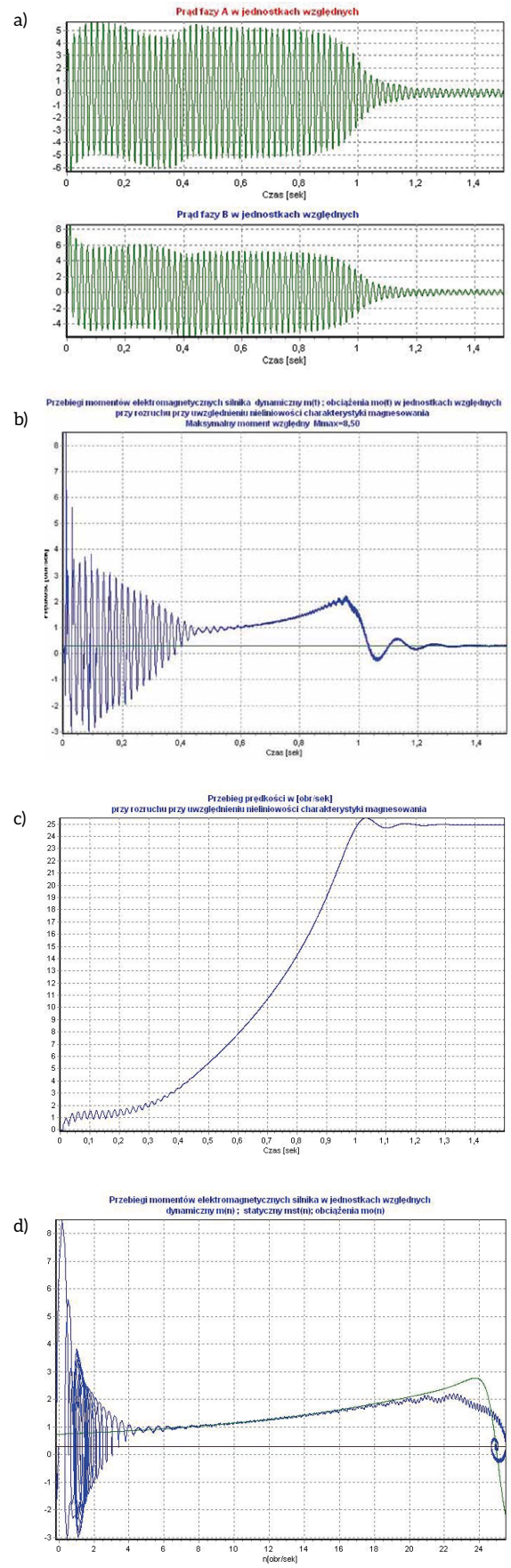
Rys. 5. Charakterystyki rozruchowe silnika indukcyjnego klatkowego SVf 400-x4: a – prądu i_a(t) i i_\beta(t) ; b – momentu elektromagnetycznego T_e(t) ; c – prędkości kątowej \omega_m(t) ; d – T_e(t) = f(\omega_m(t)) , w czasie rozruchu ( \Psi = 0, \omega_m = 0 ), przy niekorzystnej chwili załączenia napięcia
