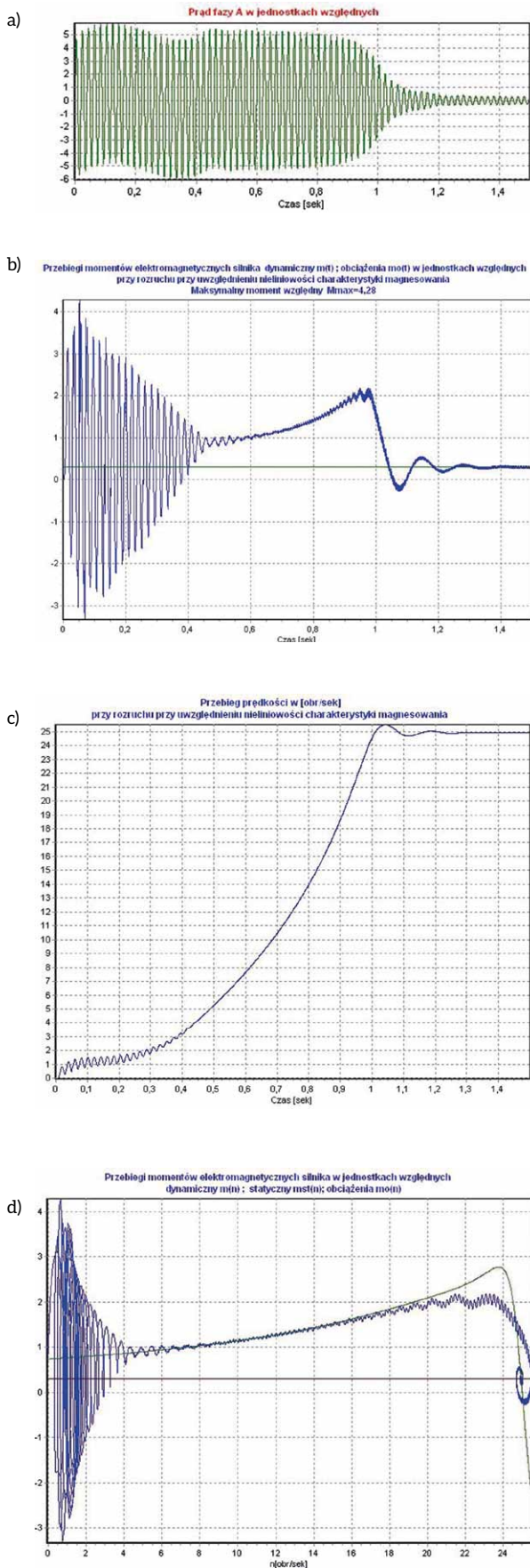
Rys. 4. Charakterystyki rozruchowe silnika indukcyjnego klatkowego SVf 400 x4: a – prądu i(t) ; b – momentu elektromagnetycznego T_e(t) ; c – prędkości kątowej \omega_m(t) ; d – T_e(t) = f(\omega_m(t)) , w czasie rozruchu ( \Psi = 0, \omega_m = 0 ) przy korzystnej chwili załączenia napięcia
