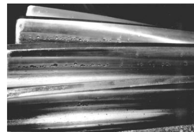
Fig. 3. Standard gear pitting damage Rys. 3. Standardowe uszkodzenie uzębienia przez pitting
