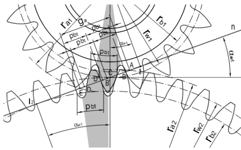
Fig. 1. Geometry of involute HCR gearing Rys. 1. Geometria ewolwentowego uzębienia HCR
