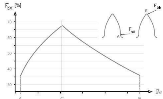
Fig. 2. Shape of the curves represents the load along the path of contact in one pair of HCR gearing teeth Rys. 2. Przebieg przenoszonego obciążenia jednej pary zębów uzębienia HCR wzdłuż odcinka
