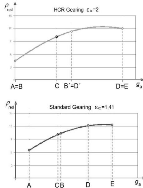
Fig. 5. Mean contact radius of curvature along the contact path Rys. 5. Zredukowany promień zakrzywienia wzdłuż odcinka przyporu
