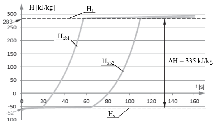
Rys. 3. Entalpia H_{xb1} i H_{xb2} w pręcie podczas przemiany fazowej w funkcji czasu dla punktów odpowiednio: x_{b1} = 0,02 i x_{b2} = 0,05
