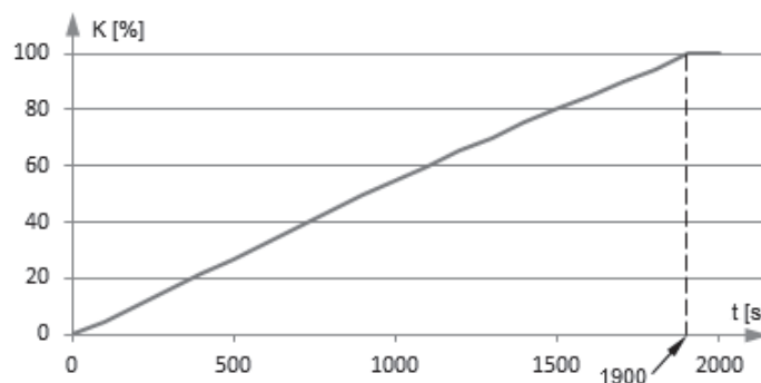
Rys. 4. Procentowe wytopienie pręta w funkcji czasu
