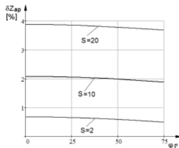
Rys. 5. Błąd \delta Z_{ap}(\varphi) dla S=2, 10 i 20 przy d_{E_{sk}} \approx 0,207 V Fig. 5. Error \delta Z_{ap}(\varphi) for S=2, 10 and 20 , for d_{E_{sk}} \approx 0,207 V
