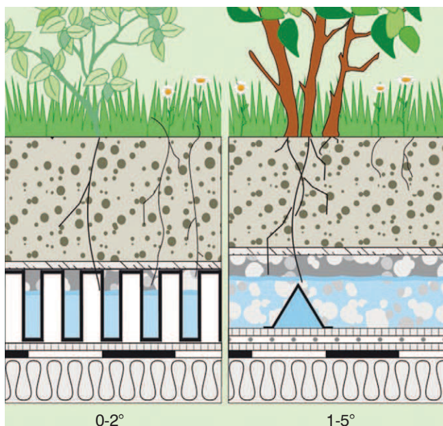
Rys. 8. Układ konstrukcyjny dachu naturalnego w zależności od nachylenia [7]
