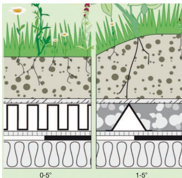
Rys. 4. Układ konstrukcyjny dachu naturalnego w zależności od nachylenia [7]
