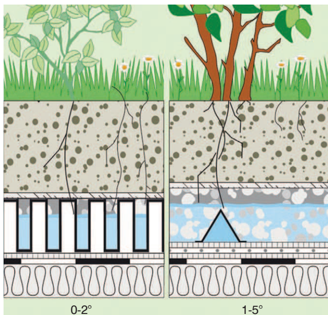
Rys. 7. Układ konstrukcyjny ogrodu na dachu w zależności od nachylenia [7]
