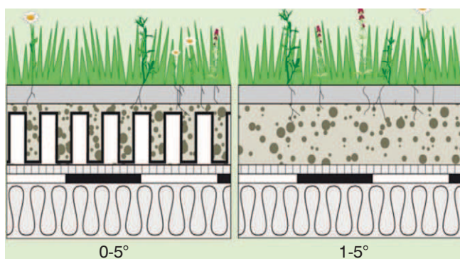
Rys. 3. Układ konstrukcyjny dachu lekkiego w zależności od nachylenia [7]
