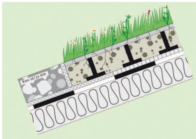
Rys. 6. Układ konstrukcyjny dachu skośnego [7]
