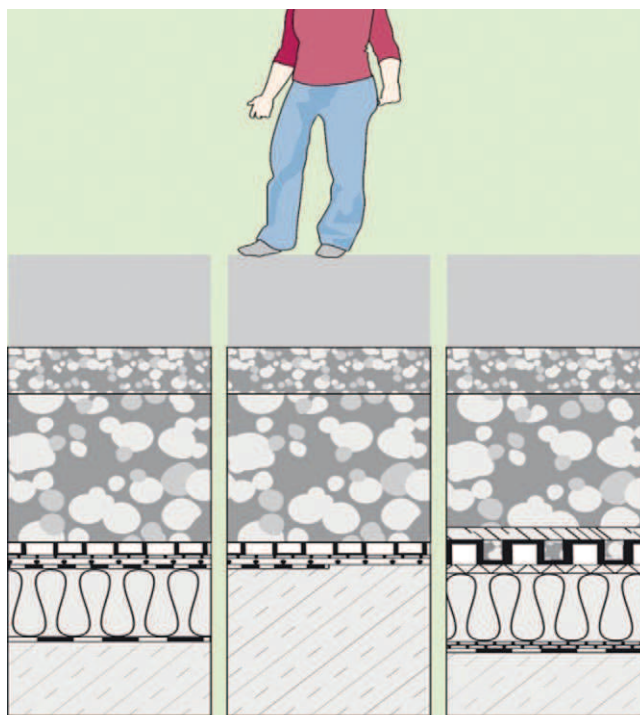
Rys. 9. Układ konstrukcyjny dachu komunikacyjnego z termoizolacją lub bez [7]
