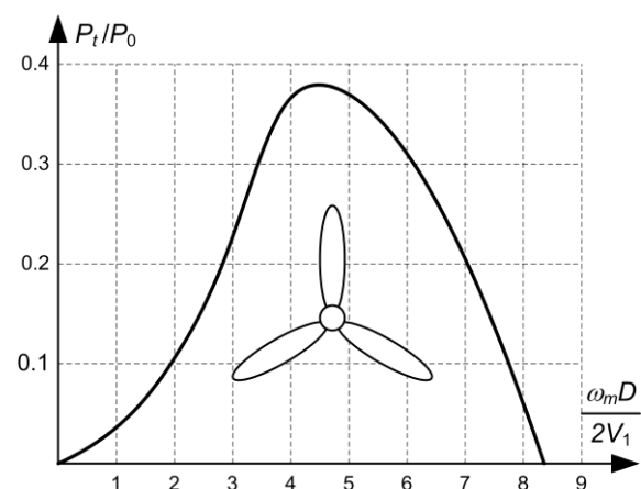
Rys. 1. Charakterystyka \frac{P_t}{P_0} = f\left(\frac{\omega_m D}{2V_1}\right) turbiny trzyłopatowej
