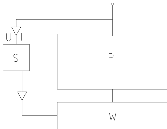
Rys. 3. Schemat blokowy zespołu elektromechanicznego odbierającego moc z turbiny wiatrowej: P – prądnicą, W – wyłączniki, S – sterownik mikroprocesorowy
