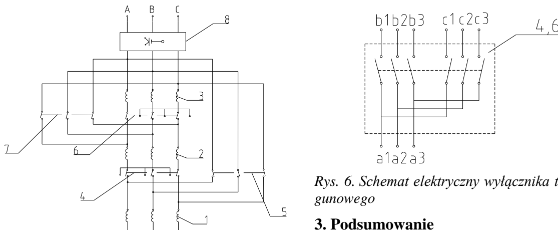
Rys. 5. Schemat połączenia uzwojenia o trzech sekcjach z wyłącznikami
