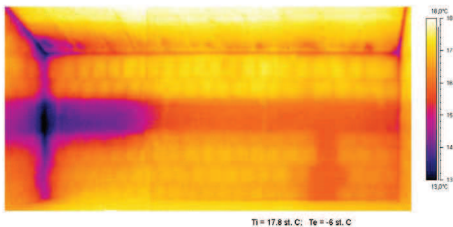
Rys. 3. Mapa rozkładu temperatury na powierzchni ściany dwuwarstwowej
