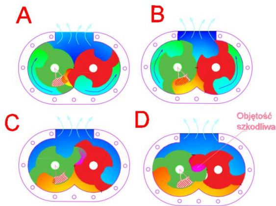
Rys. 3. Cykl pracy silnika pneumatycznego pracującego w cyklu odrotnym do cyklu sprężarki zębatej
