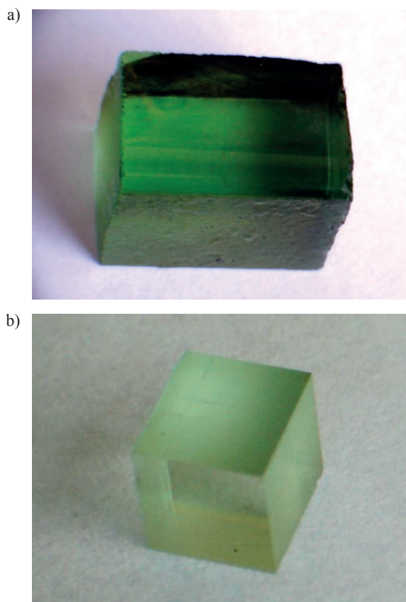
Rys. 1. Fotografia badanego szkła ELG: a) bryła szkła po wytopie, b) przykładowa próbka szkła ELG o wymiarach 4 \times 4 \times 5 mm przygotowana do badań.
