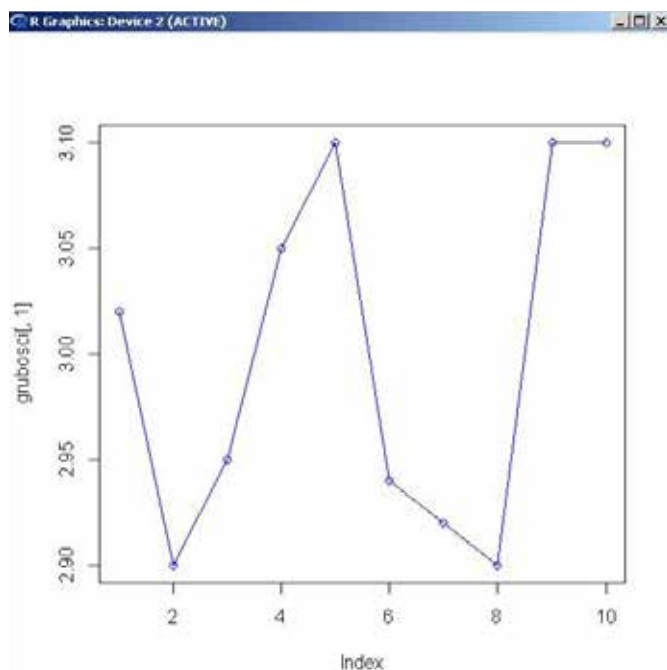
Rys. 8. Wygenerowany w programie R wykres dla czasu anodowania 10 minut (próbka nr 4). Na osi x numer kolejnego pomiaru, na osi y wartość grubości powłoki anodowanej w [µm]
